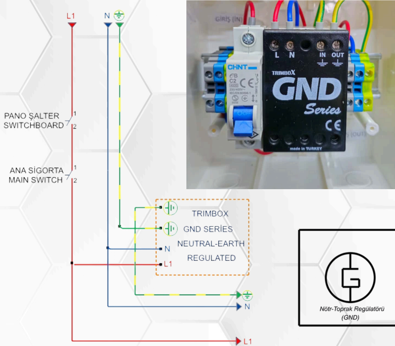
TRIMBOX NÖTR-TOPRAK REGÜLATÖRÜ GND SERIES BAĞLANTI ŞEMASI
